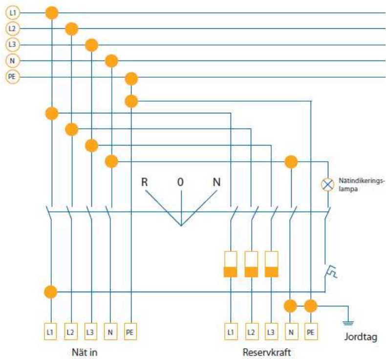
Figur 6 Reservkraft TN-S
