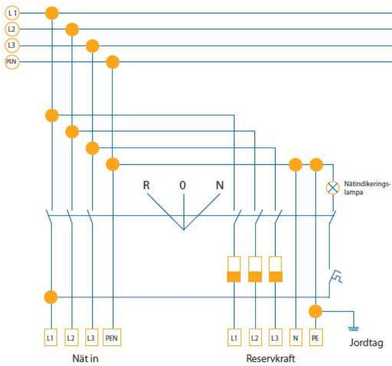
Figur 7 Reservkraft TN-C
